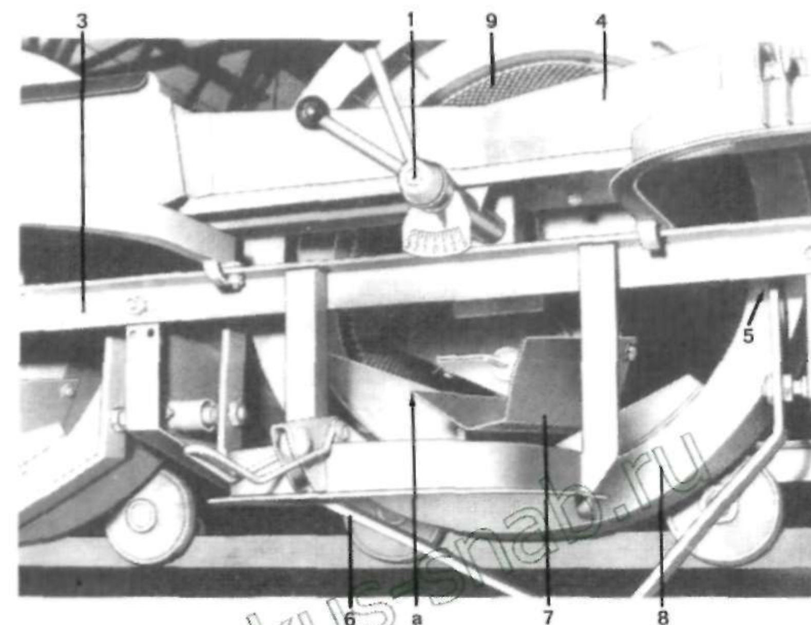
Рис. 22: Элементы обслуживания и работы триера
