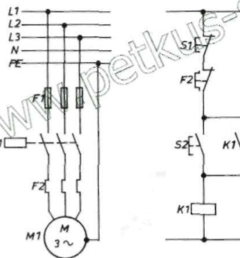
Рис. 14: Электрическая схема
