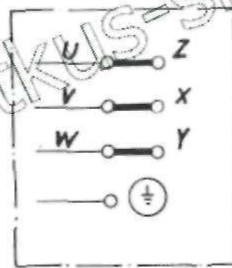
Рис. 9 схема включения \Delta при 220 в
