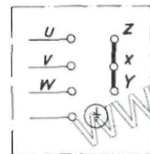
Рис. 8 схема включения \lambda при 380 в
