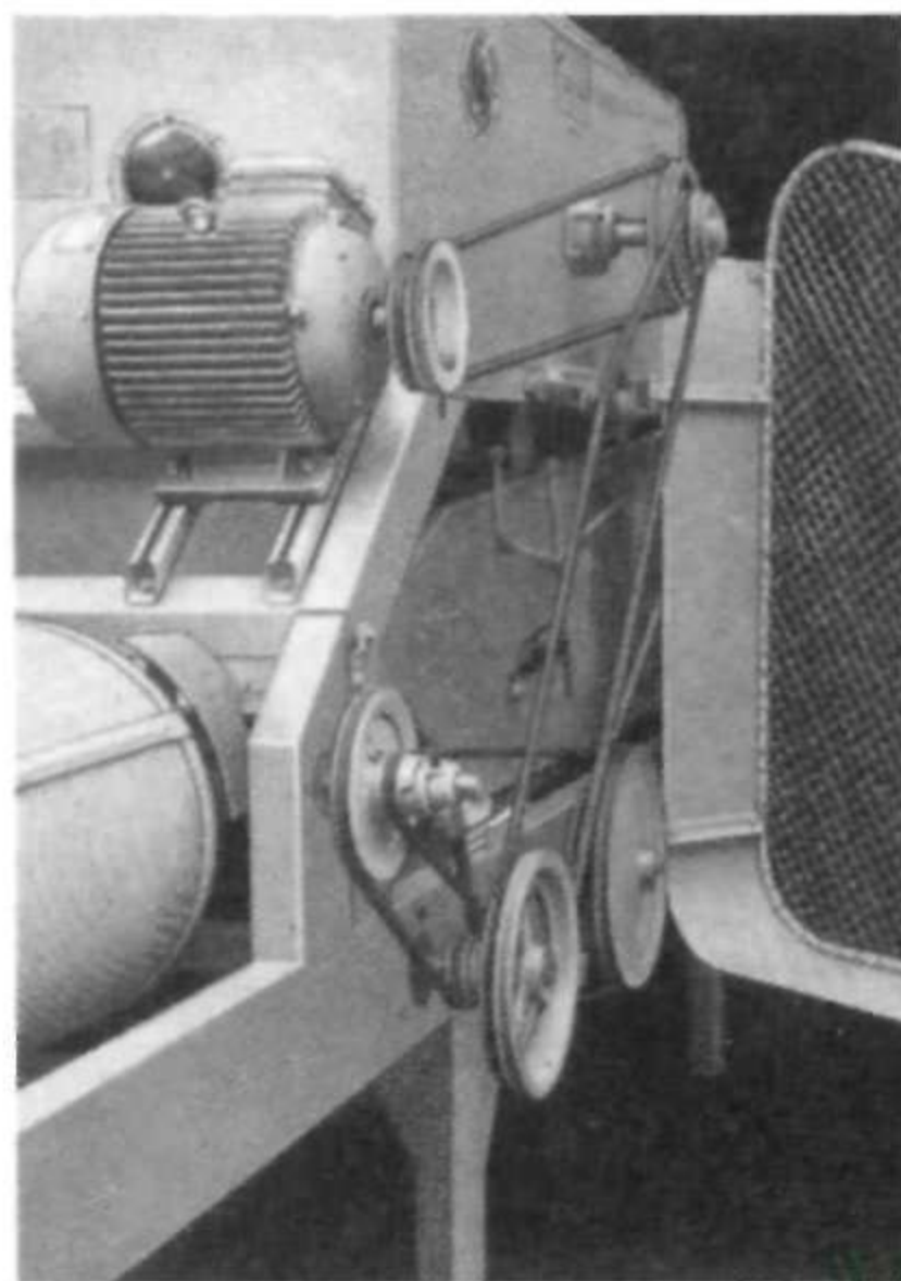
Рис. 3: Поворотная защитная решетка
